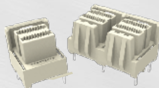
Serie 900 (SMT) (1x1 Puerto, 1x2 Puerto) Impedancia: 85Ω
